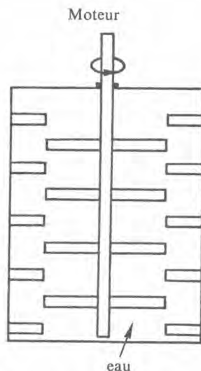
3- 1 : Schéma de principe d'une expérience de Joule.
