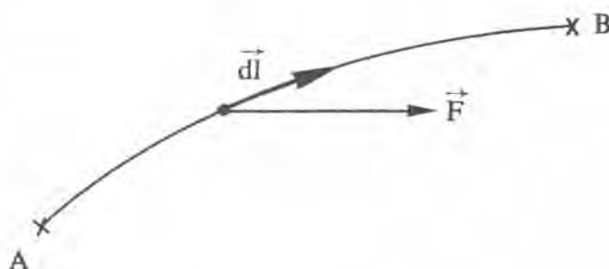
2- 1 : Calcul du travail de la force \vec{F} .
