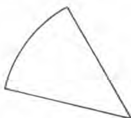
un secteur saillant est convexe
