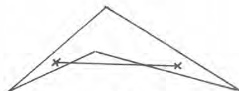
quadrilatère non convexe
