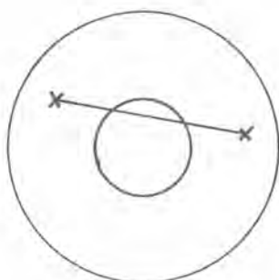
la couronne n'est pas convexe
