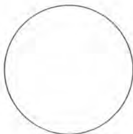
le disque est convexe
