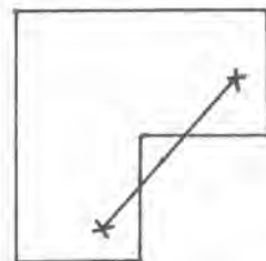
ce domaine n'est pas convexe
